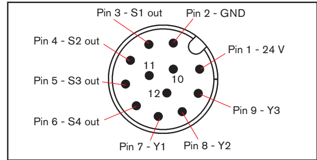
(12-poliger Rundsteckverbinder M12 x 0,75 - male nach IEC 61076-2-101 — Blick auf Steckerstifte)
